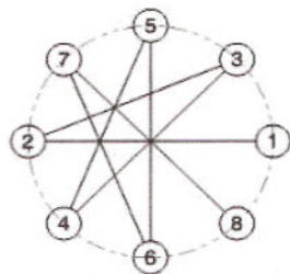
8 LUG BOLT PATTERN
